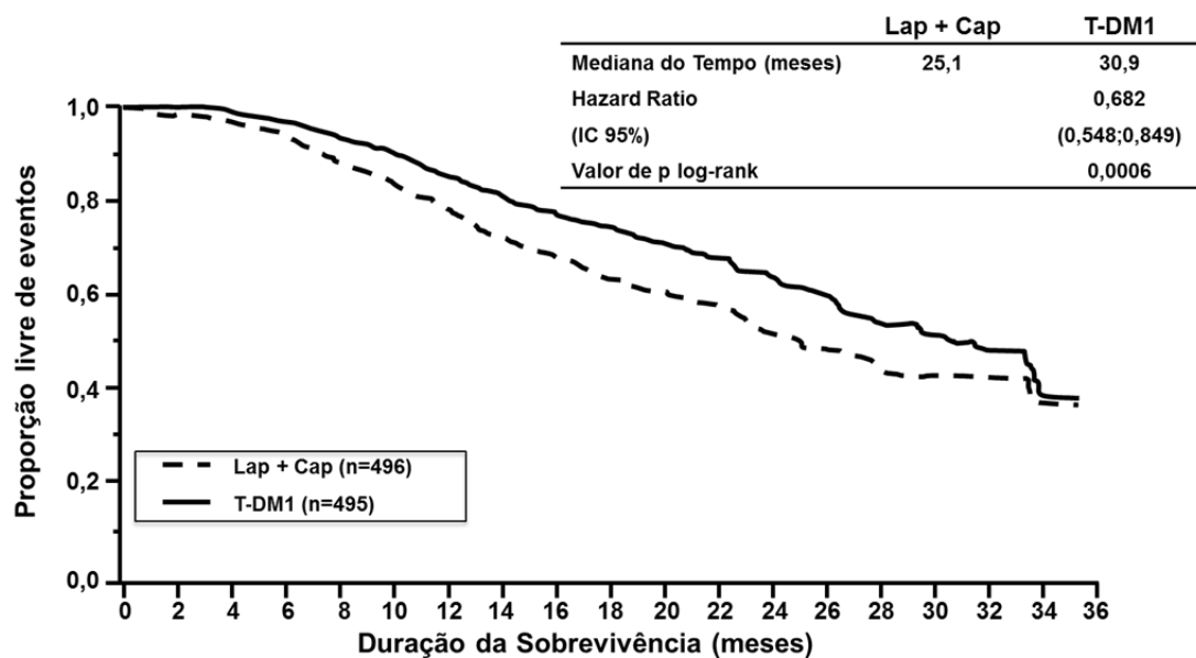
Figura 4 Curva de Kaplan-Meier da sobrevivência global
