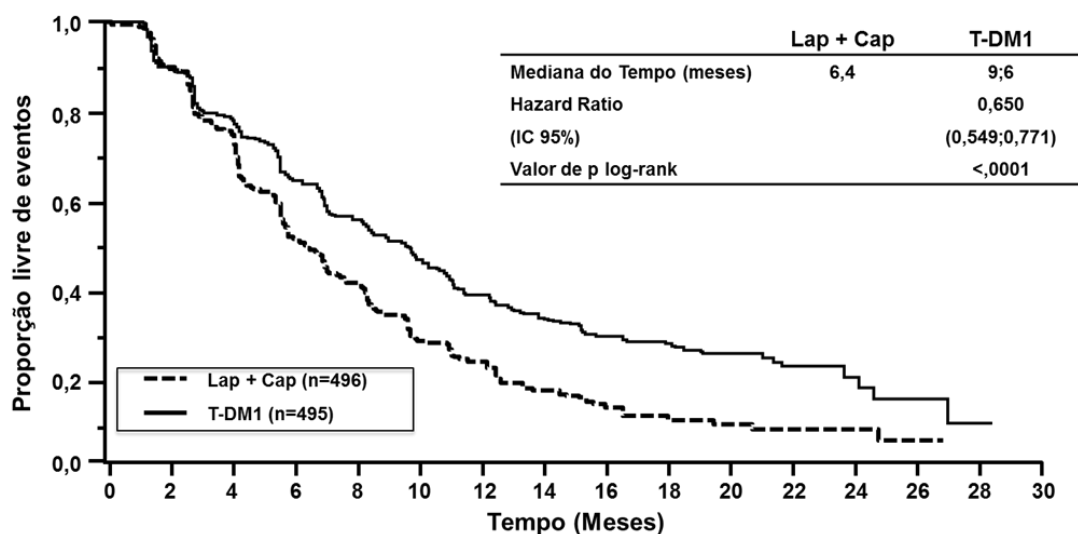
Figura 3 Curva de Kaplan-Meier da sobrevivência livre de progressão, avaliada pela IRC
