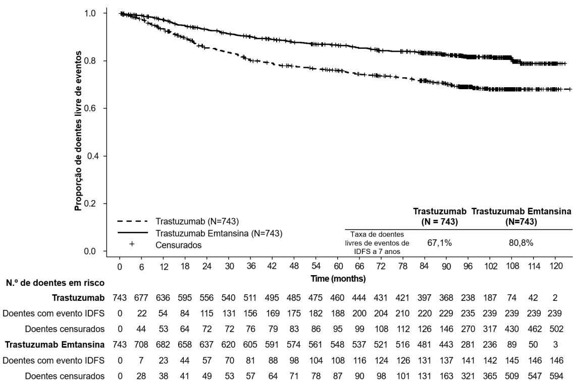
Figura 2 Curva de Kaplan-Meier da sobrevivência global no KATHERINE (análise atualizada)
